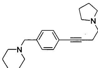
1-[4-(4-Pyrrolidin-1-yl-but-1-ynyl)-benzyl]-piperidine
