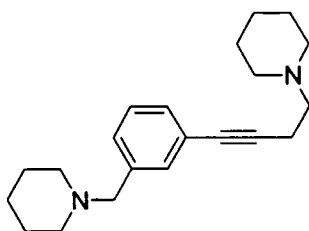
1-[3-(4-Piperidin-1-yl-but-1-ynyl)-benzyl]-piperidine
