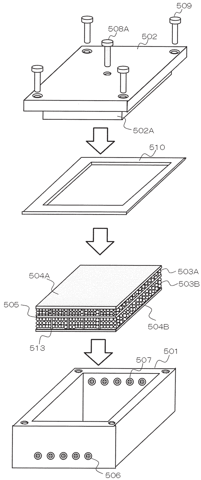
FIG.23
