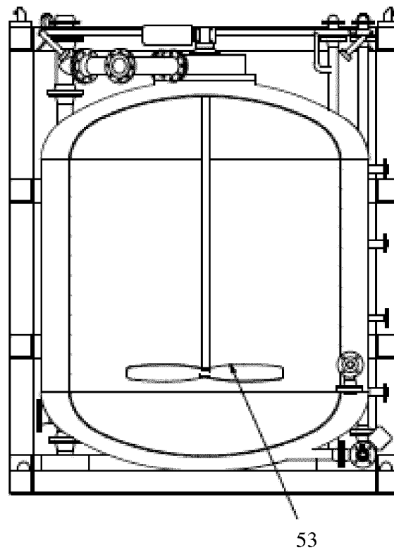
Fig. 7 (C-C)
