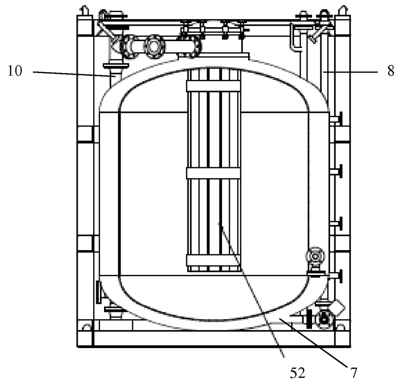
Fig. 6 (C-C)
