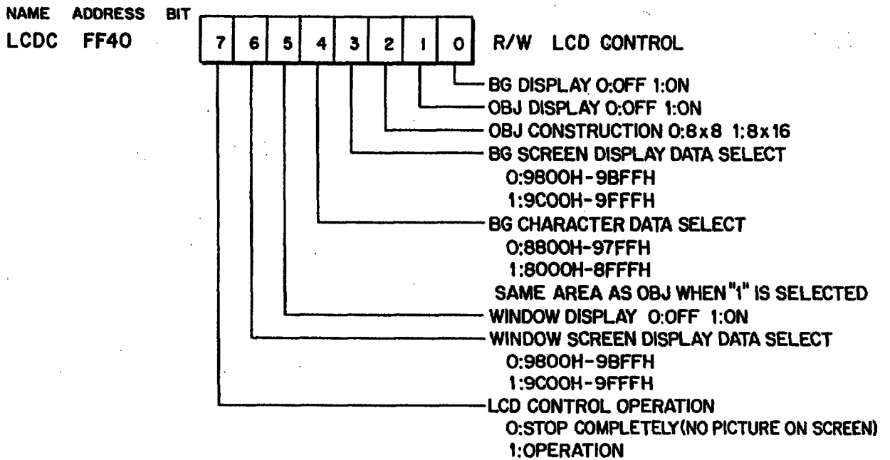
FIG. 15A LCD DISPLAY REGISTER
