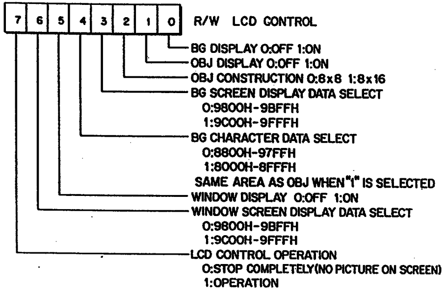
FIG. 15A LCD DISPLAY REGISTER
