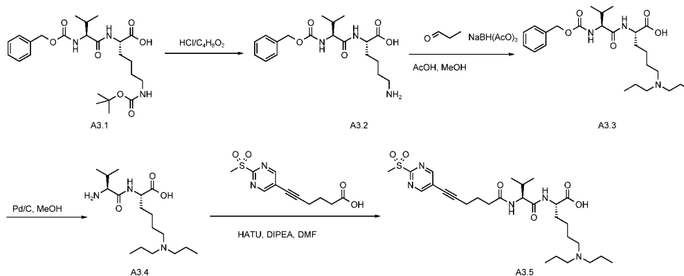
方案 3: 化合物 A 3.5 的合成路线
