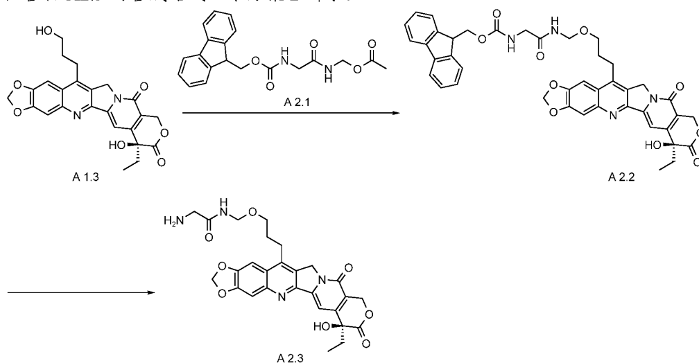
方案 2: 化合物 A2.3 的合成路线
