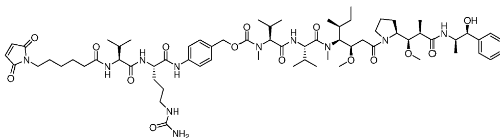
MC-VC-PABC-MMAE
