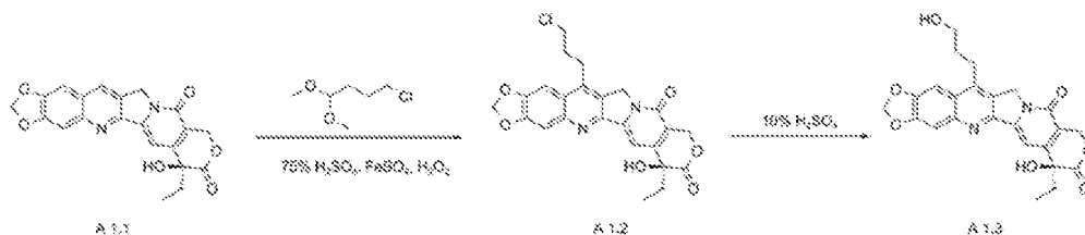
方案 1: 活性化合物 A1.3 的制备
