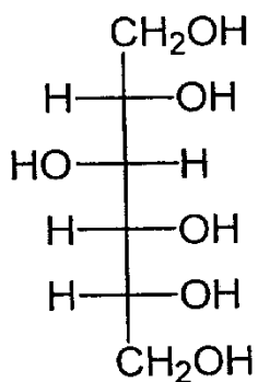
sorbitol
