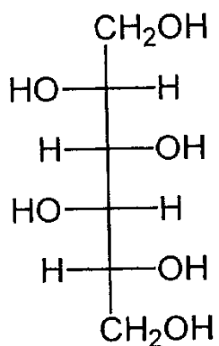
iditol
