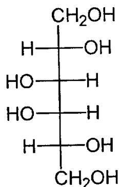
galactitol
