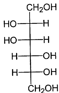
mannitol
