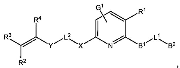
Id
