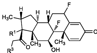
(PVIIb).
