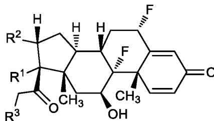
(PVIII).
