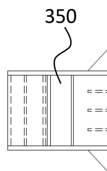
FIG. 28B (VIEW E1-E1)
