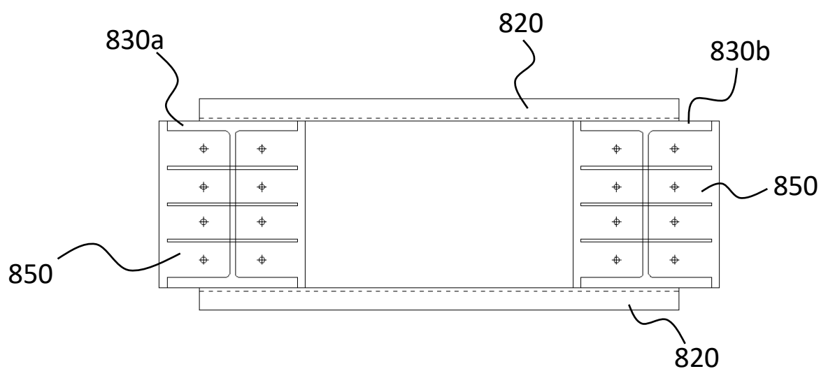
FIG. 48 (VIEW E2-E2)
