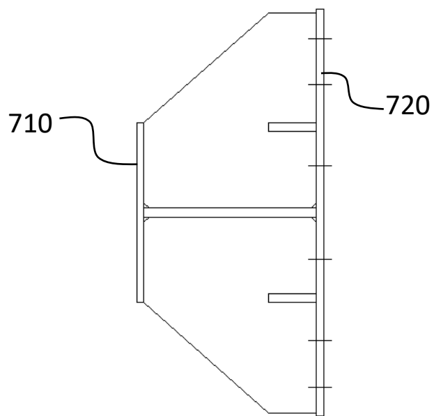
FIG. 43 (VIEW D2-D2)
