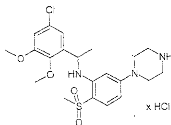
PRX-07034
