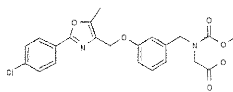
BMS-687453
