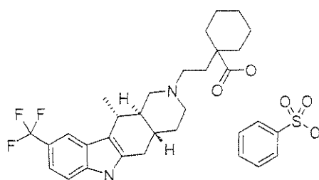
AMG-071
