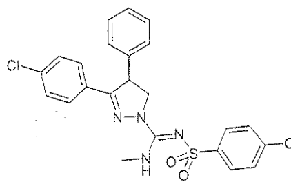
SLV-319
