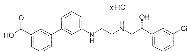
solabegron
