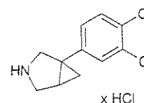
DOV-21947
