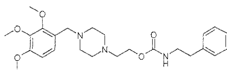
ST-3473
