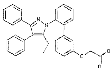
BMS-309403
