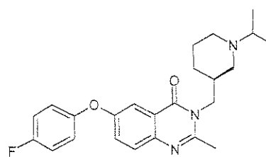
YIL-781
