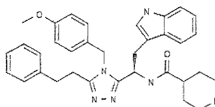
JMV-2951
