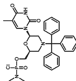
Thymine morpholino monomer
