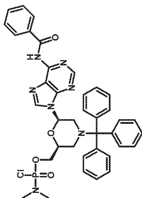
Adenine morpholino monomer
