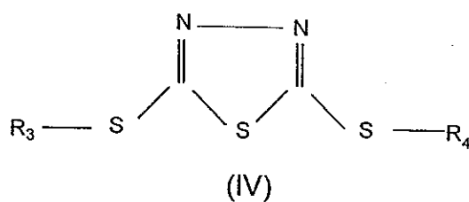
2,5-bis(hydrocarbylthio)-1,3,4-thiadiazole
