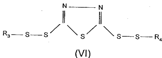
2,5-bis(hydrocarbyldithio)-1,3,4-thiadiazole
