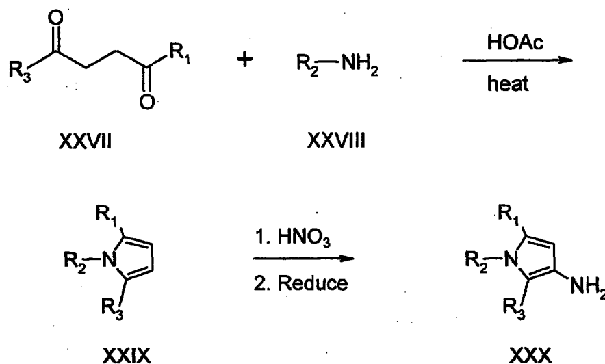
Scheme VI
