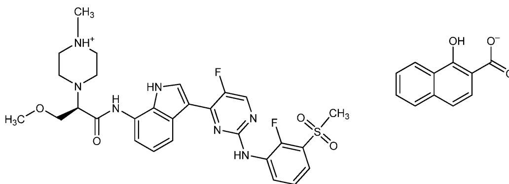
Formula (Ia).
