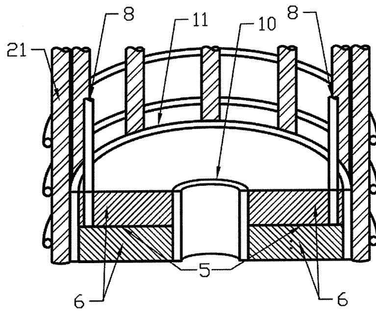
FIG. 6C
