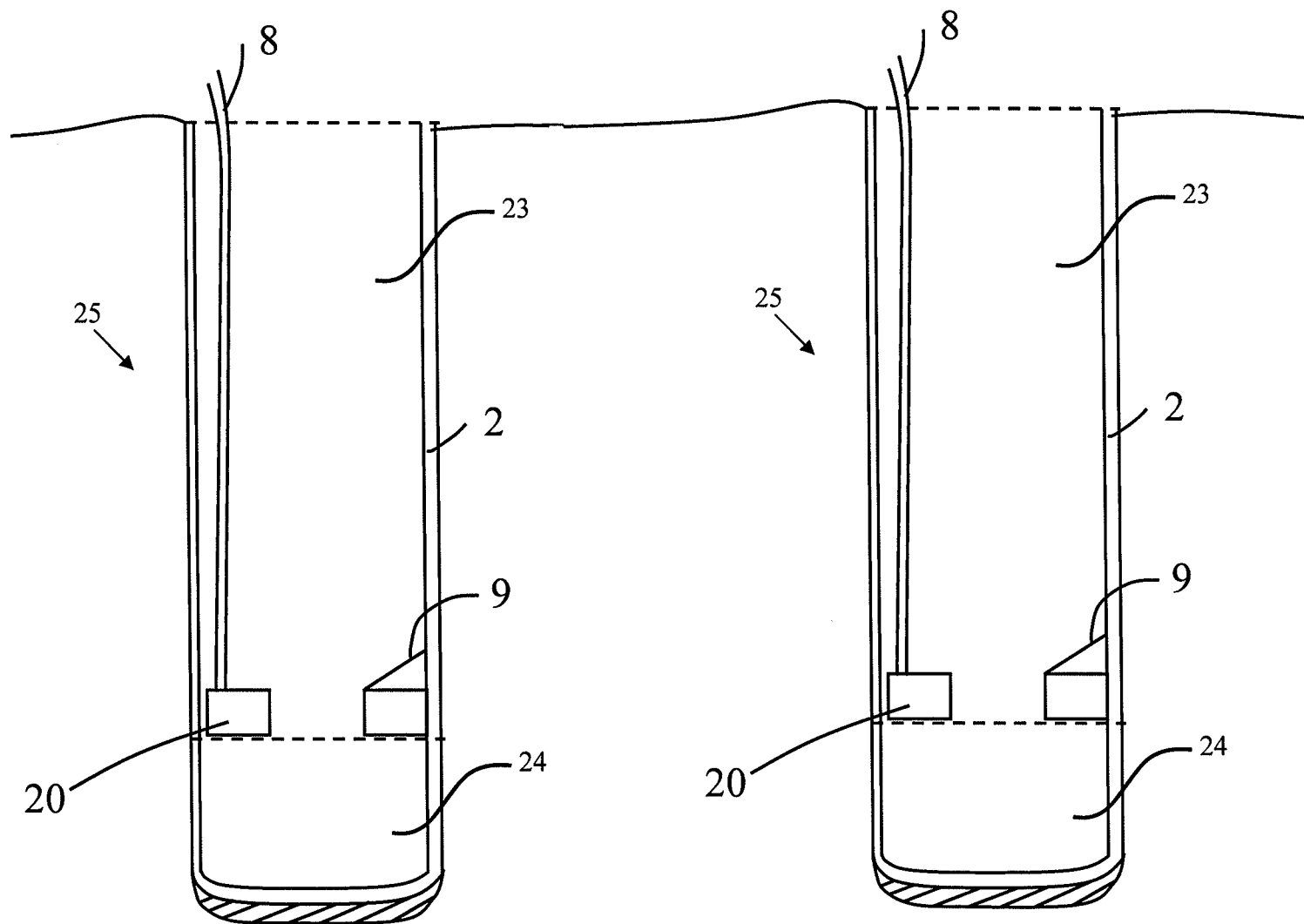
FIG. 7
