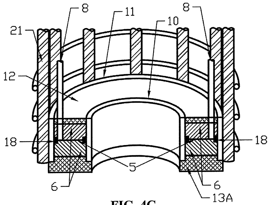
FIG. 4C
