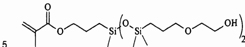
iSiMAA3-Me
