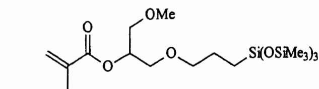
iSiMAA3-Me
