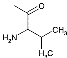
valyl
