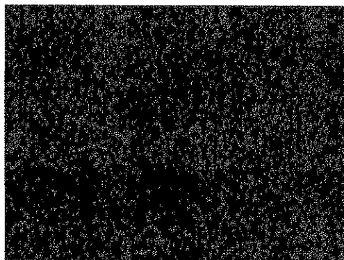
Co Ka1
