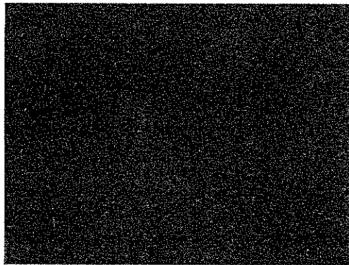
Ru La1
