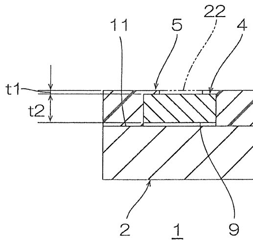
FIG. 4B(Comparative Example)
