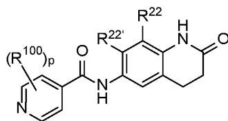
(IV-D)
