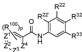
(IV-B)
