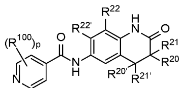
(IV-C)
