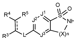
Formula II-4
