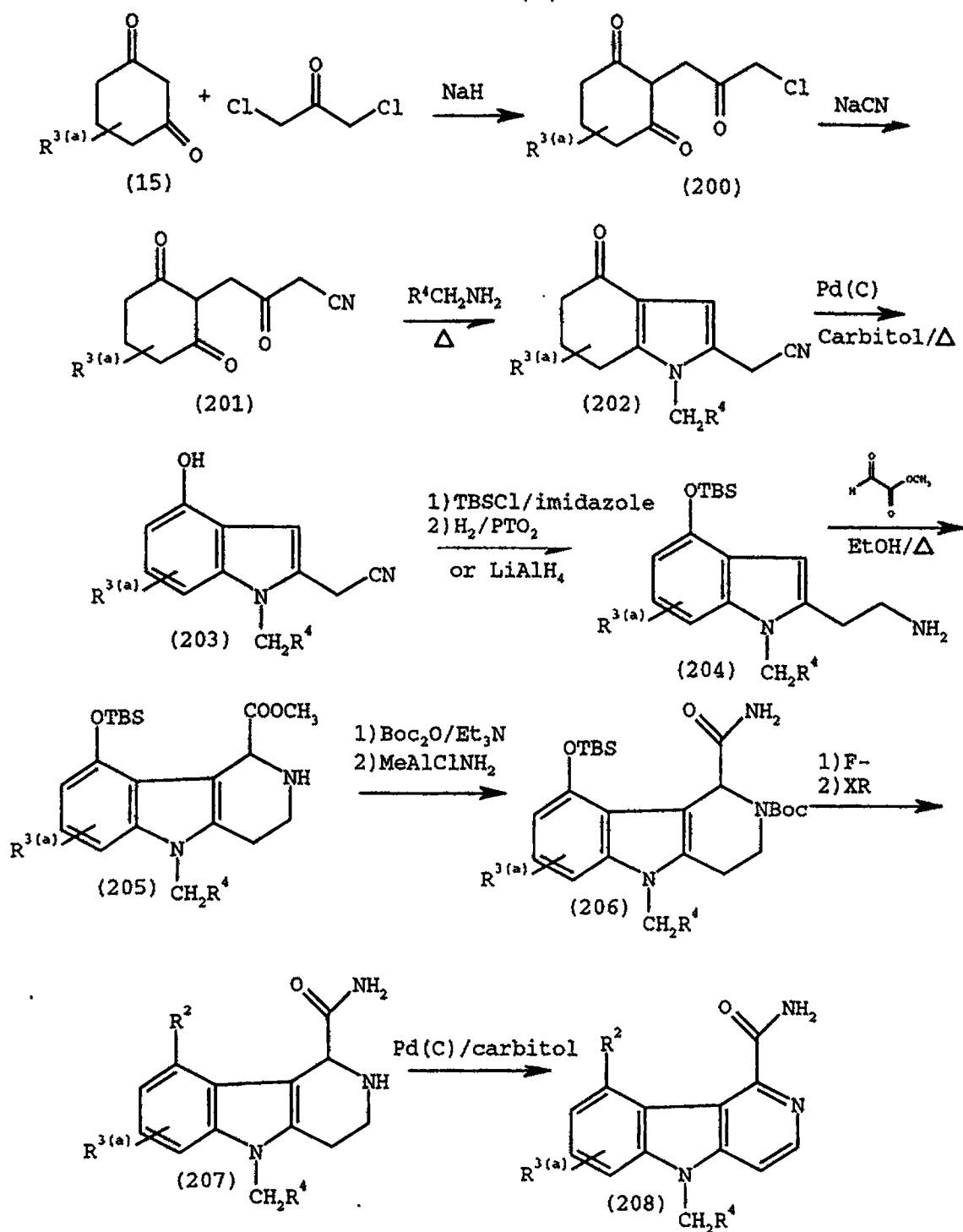
Scheme V(d)
