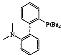
'B_A_B
