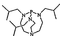
VerK_B
