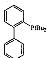
'But_B
