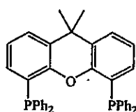
XANTPHOS
