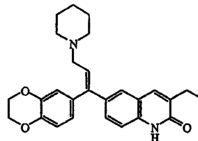
intermediate 42 (Z isomer)
