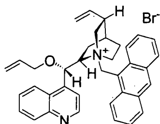
(-)-O-(9)-allyl-N-(9-anthracenylmethyl)cinchoninium bromide
