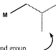
isobutyl end group
