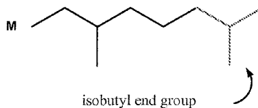
isobutyl end group
