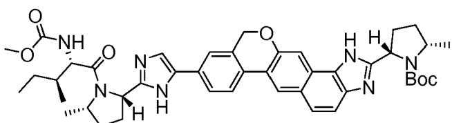
tert-butyl (2S,5S)-2-[9-(2-((2S,5S)-1-[N-(methoxycarbonyl)-L-isoleucyl]-5-methylpyrrolidin-2-yl)-1H-imidazol-5-yl)-1,11-dihydroisochromeno[4',3':6,7]naphtho[1,2-d]imidazol-2-yl]-5-methylpyrrolidine-1-carboxylate
