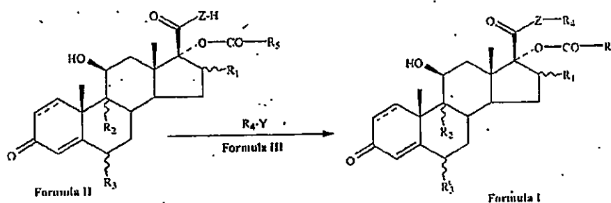
Scheme-I
