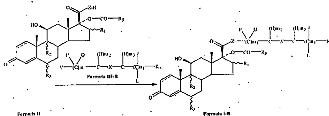
Scheme-IV
