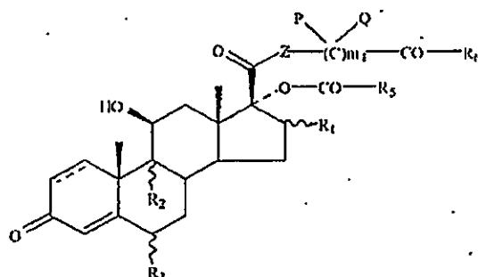
Formula I-A
