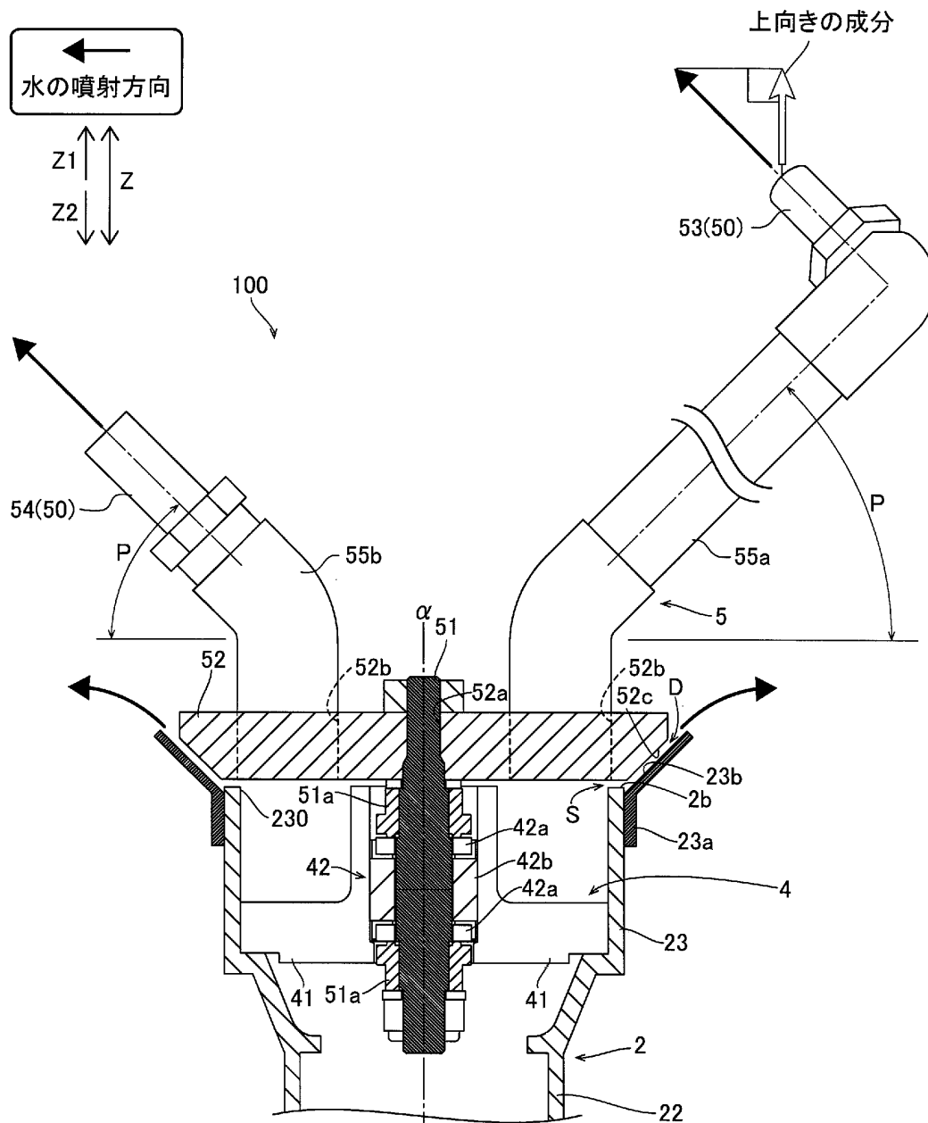
500-500断面
