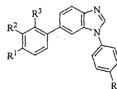
Formula VIIb
