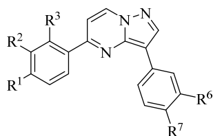
Formula Va
