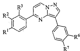
Formula Va
