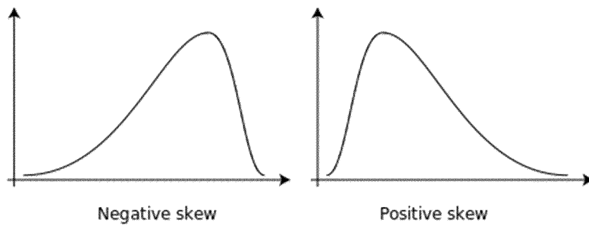
Fig. 1b Skewness
