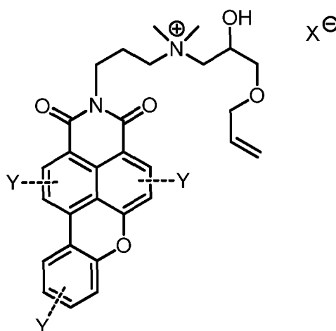
(S-NDMAPBXA-DCI-HAPQ)
