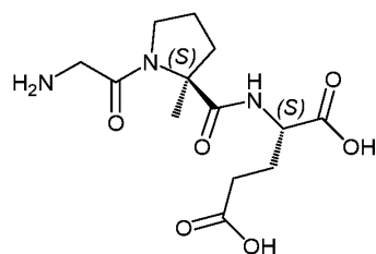
(Ia) (trofinetide),
