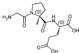
(Ia) (trofinetide),
