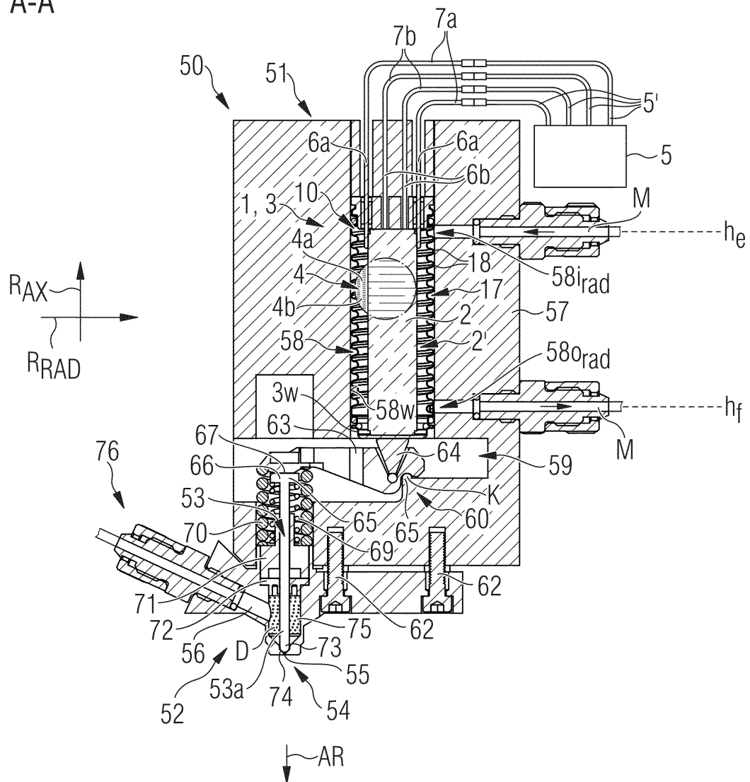
FIG 2 A-A
