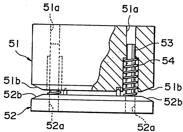
D-D SECTION
