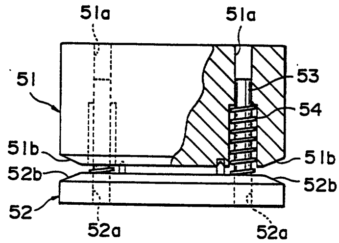
D-D SECTION
