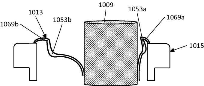
SECTION I-I FIG. 10b
