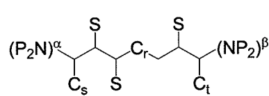
Structure AF
