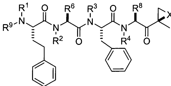
(IV)
