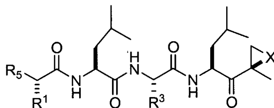
(VIII)
