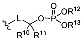
(IXa)
