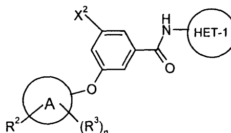
(VI)
