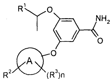
(XI)
