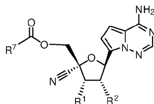
Formula VI.
