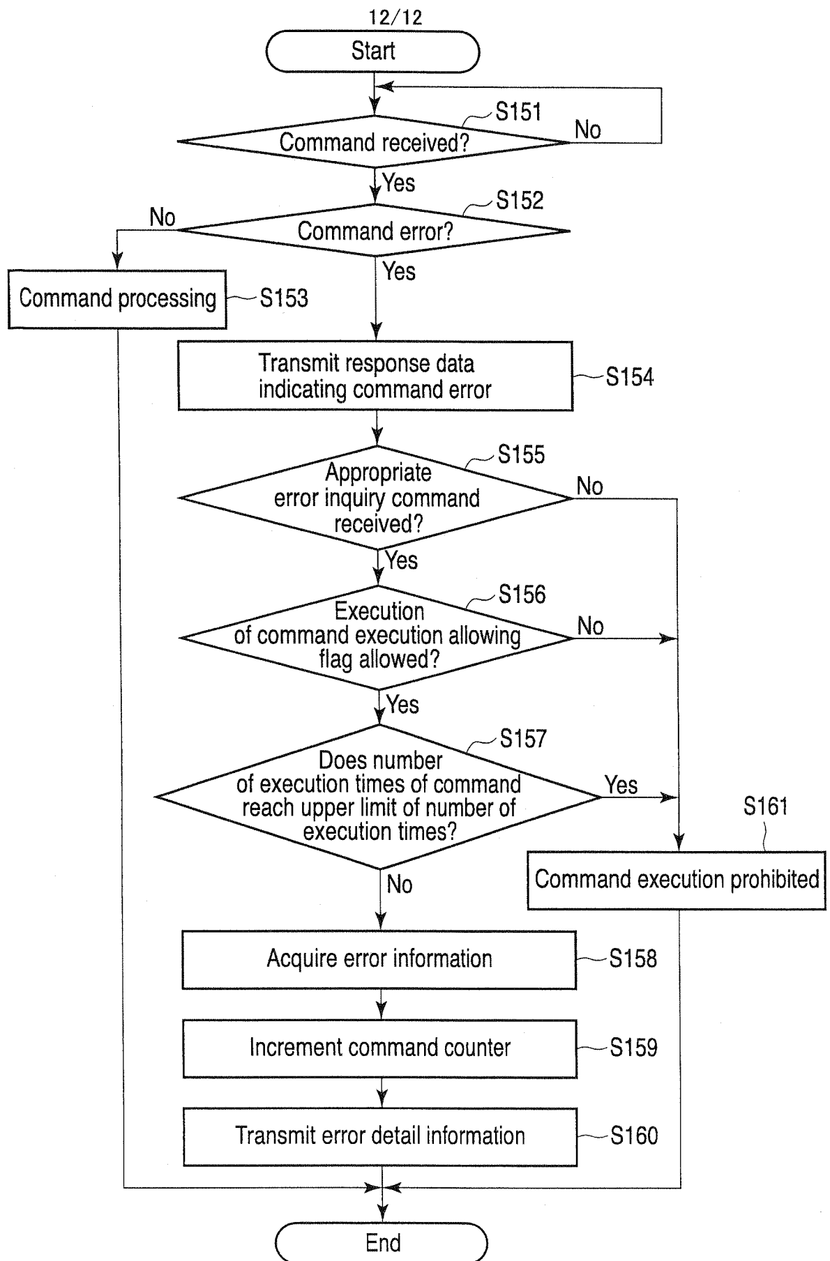
FIG. 18
