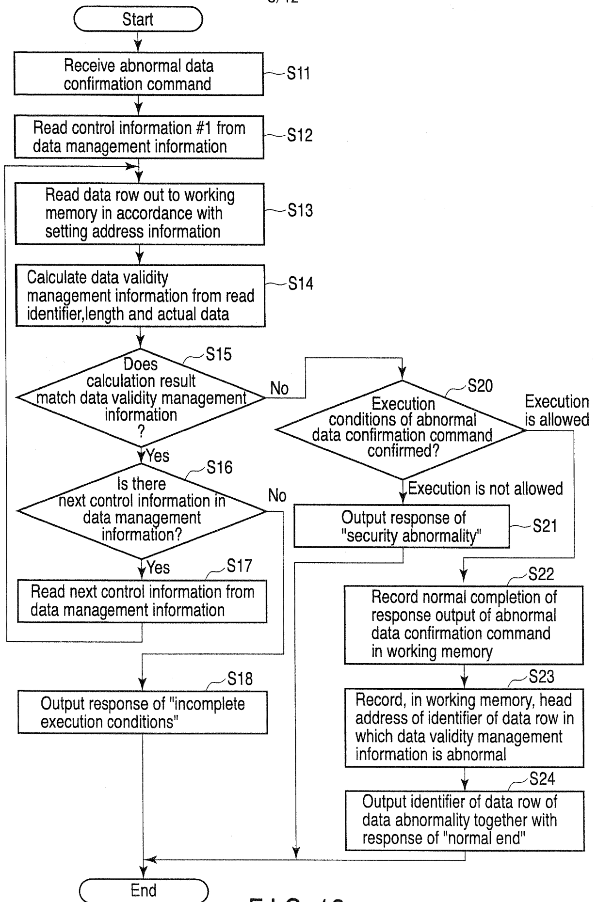
FIG. 12
