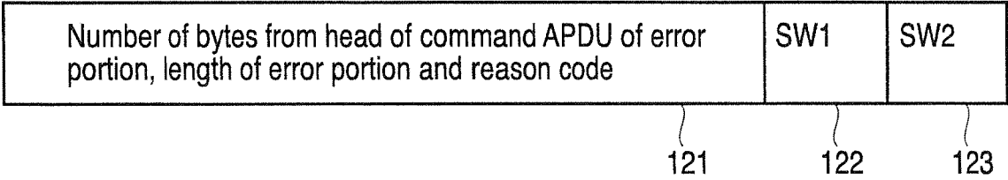
FIG. 15
