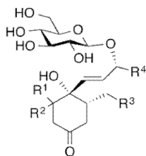
化学式 (6)
