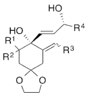
化学式 (9)
