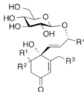
化学式 (15)
