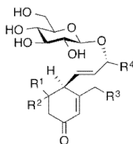
化学式(12)
