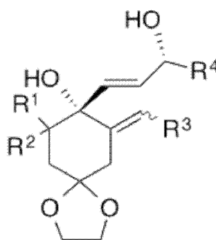
化学式 (9)
