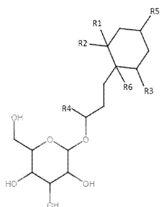
化学式 C
