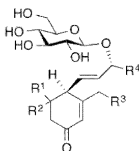
化学式(12)
