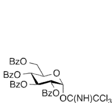
化学式 (10)
