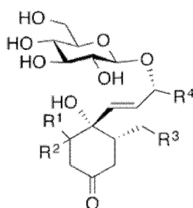
化学式 (6)
