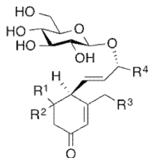
化学式(12)
