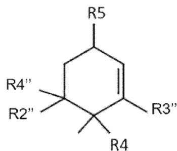
化学式 (4)
