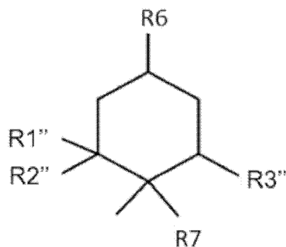
化学式(5)
