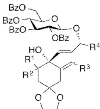
化学式(11)
