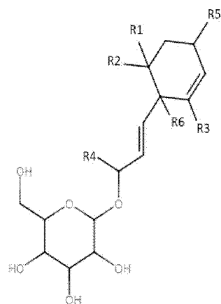
化学式 B
