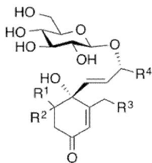
化学式(15)
