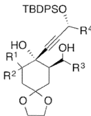
化学式 (8)
