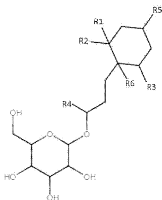
化学式 C
