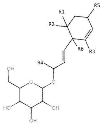
化学式 B
