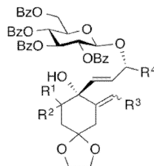
化学式 (11)
