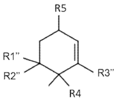
化学式(4)
