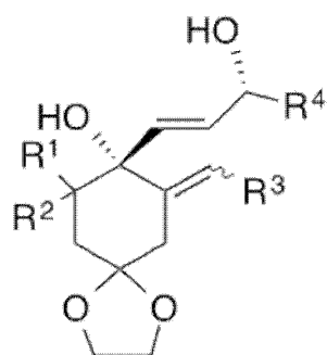
化学式 (9)
