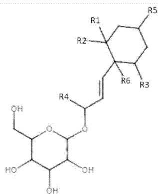
化学式 A
