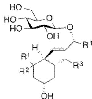
化学式(13)
