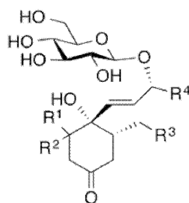
化学式 (6)
