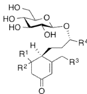
化学式(14)
