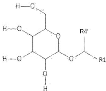
化学式 (1)
