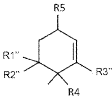
化学式(4)
