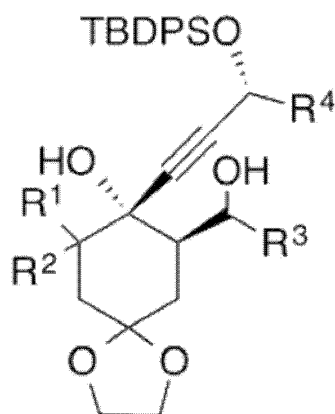
化学式 (8)
