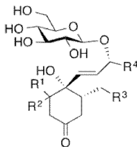
化学式 (6)
