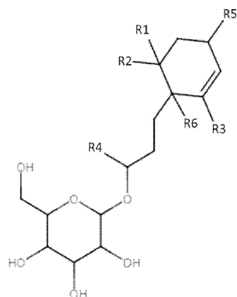
化学式 D
