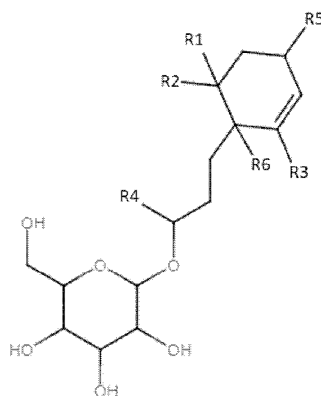
化学式 D
