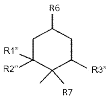
化学式 (5)
