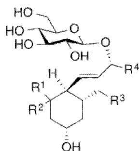
化学式(13)
