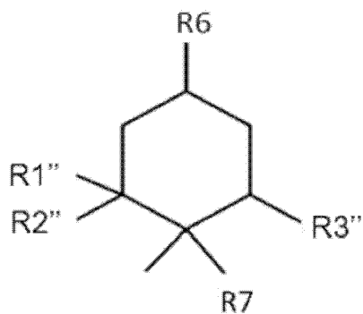
化学式(5)
