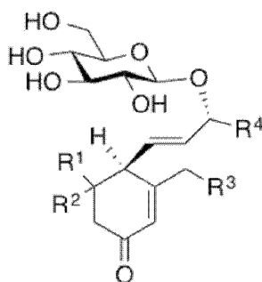
化学式(12)
