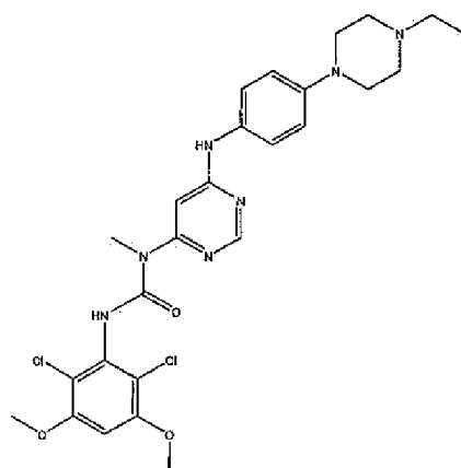
BGJ398
