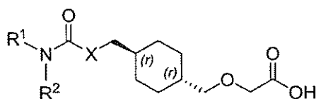
(1 r ,4 r )- or trans - mesoisomer
