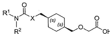
(1 s ,4 s )- or cis - mesoisomer
