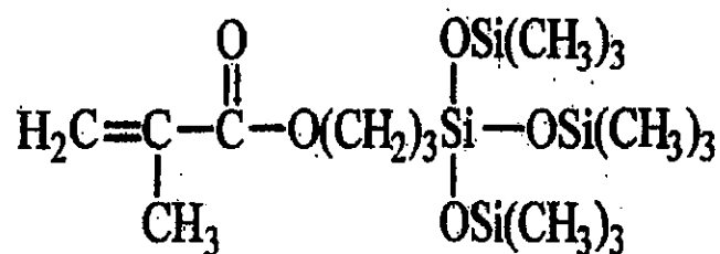
Tris
