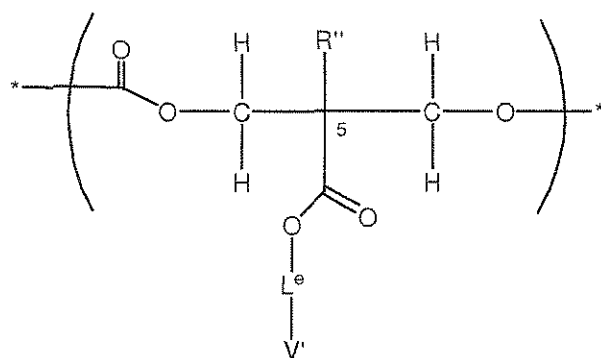
(3),
