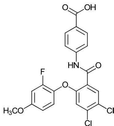
4-(4,5-dichloro-2-(2-fluoro-4-methoxyphenoxy)benzamido)benzoic acid;
