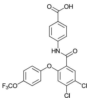
4-(4,5-dichloro-2-(4-(trifluoromethoxy)phenoxy)benzamido)benzoic acid;
