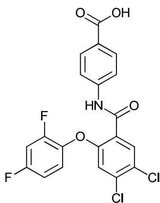
4-(4,5-dichloro-2-(2,4-difluorophenoxy)benzamido)benzoic acid;
