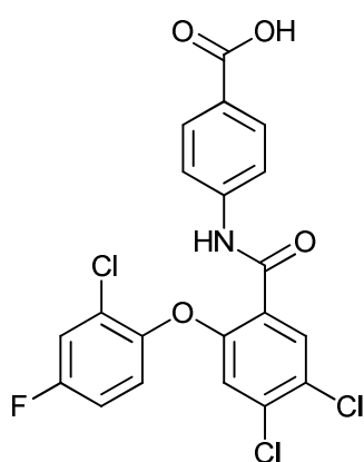
4-(4,5-dichloro-2-(2-chloro-4-fluorophenoxy)benzamido)benzoic acid;
