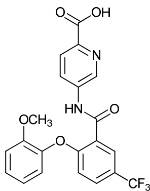
5-(2-(2-methoxyphenoxy)-5-(trifluoromethyl)benzamido)picolinic acid;
