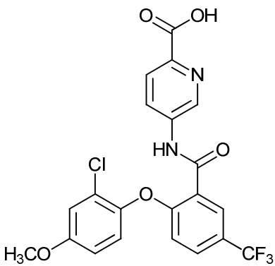
5-(2-(2-chloro-4-methoxyphenoxy)-5-(trifluoromethyl)benzamido)picolinic acid;
