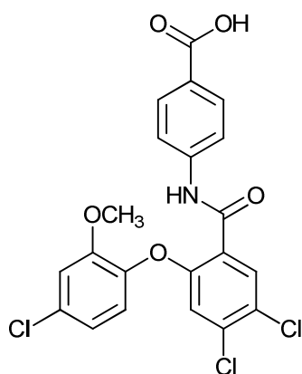
4-(4,5-dichloro-2-(4-chloro-2-methoxyphenoxy)benzamido)benzoic acid;
