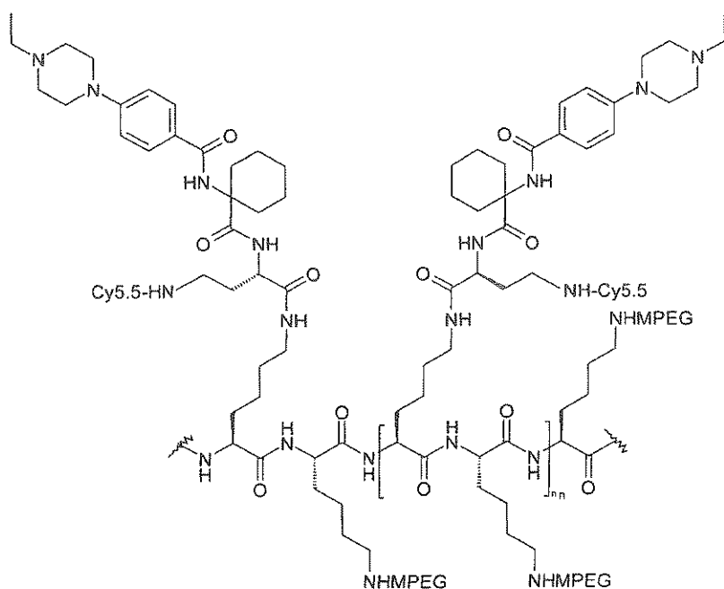
(Scheme 20)
