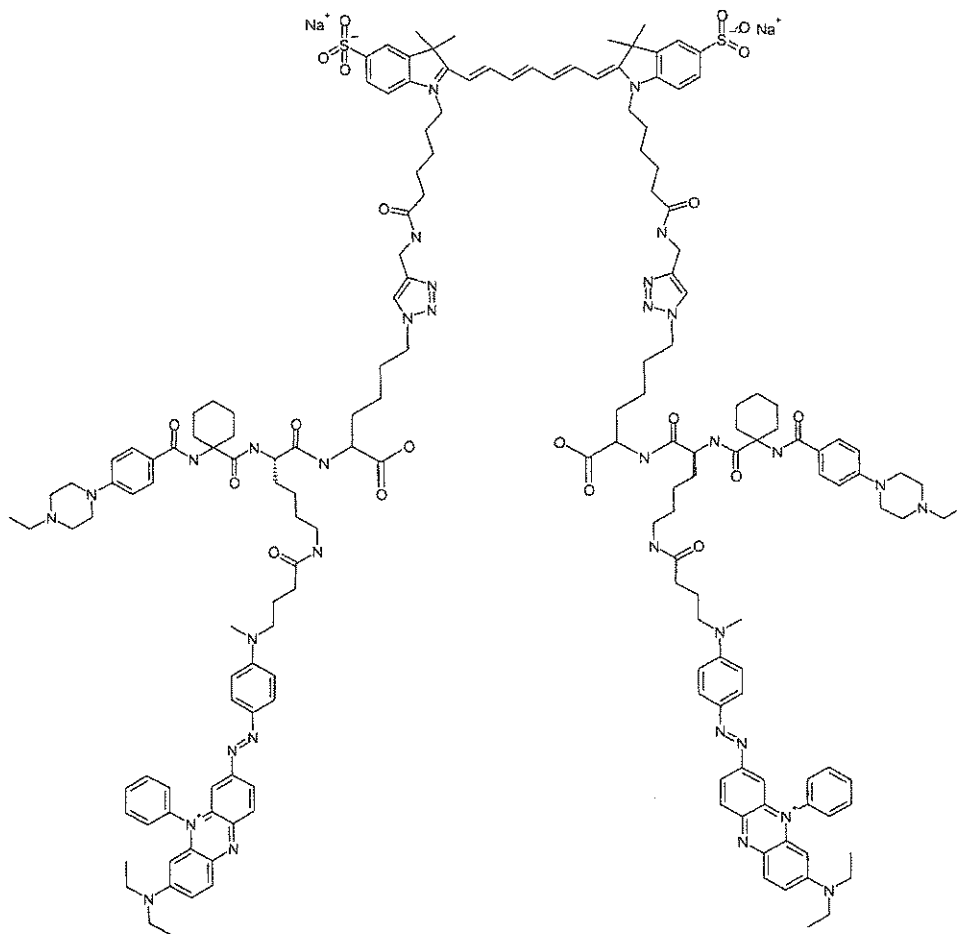
(Scheme 18).
