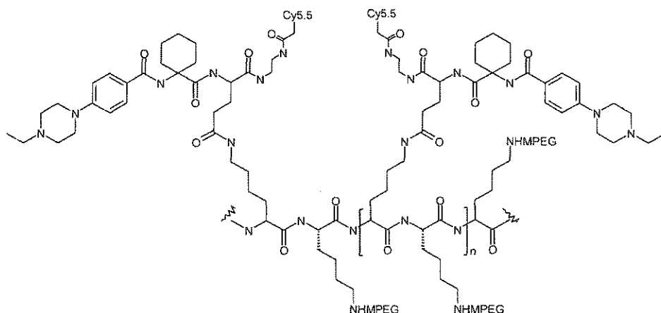
(Scheme 19)
