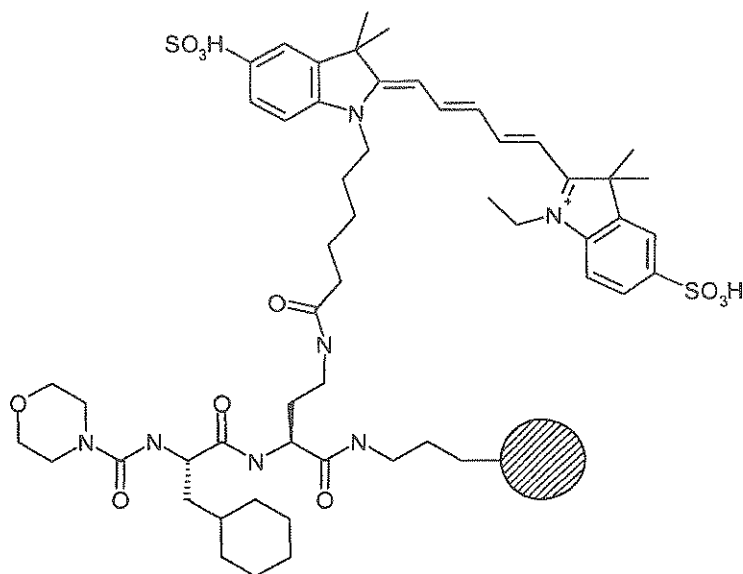
(Scheme 15).
