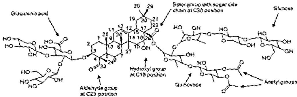
SAPONIN A
