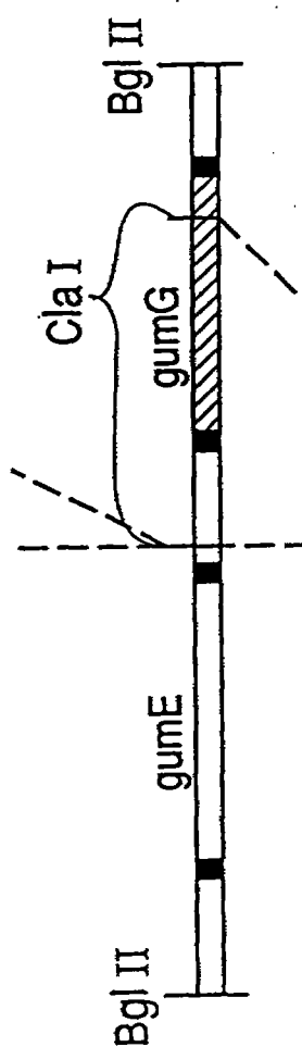
FIG. 7b pSIBgl ΔCla
