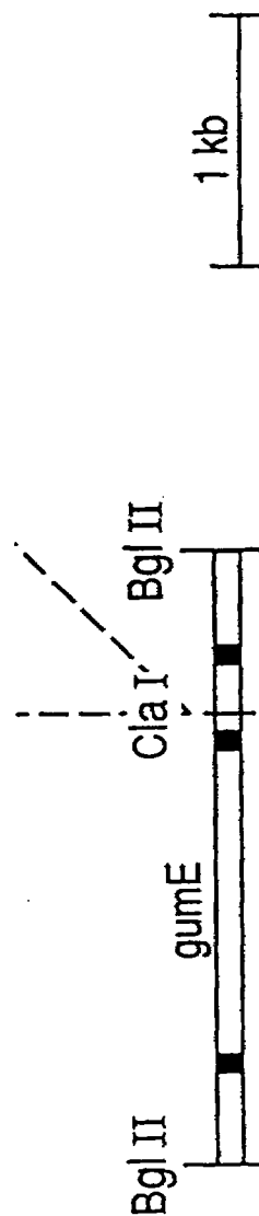
FIG. 7c pSIBgl ΔCla2
