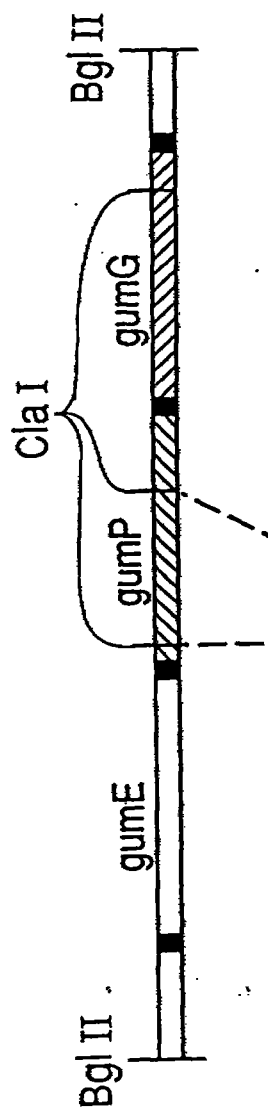
FIG. 7a pSIBgl
