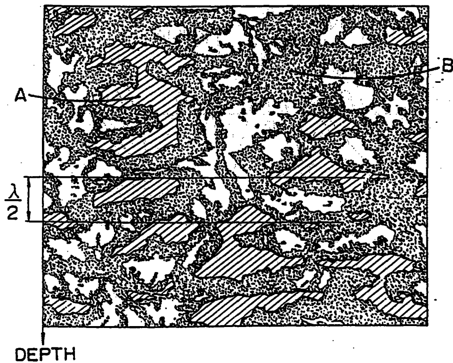
FIG. 5(b) FREQUENCY : 50KHz
